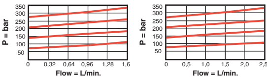
泄压曲线
