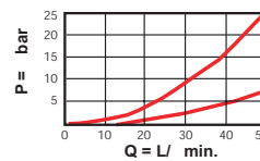
DRBO 压损
